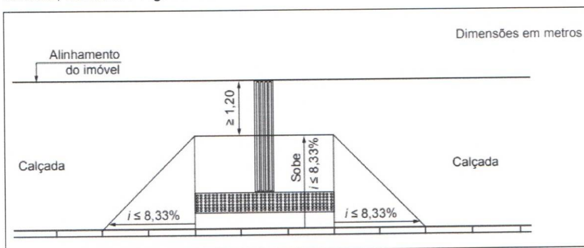
Figura 01 - Rebaixamento de Calçada TIPO 1
