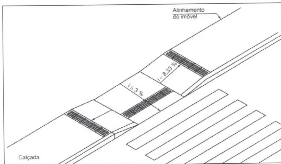
Figura 02: Rebaixamento de Calçada TIPO 2
